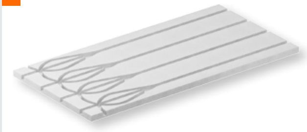
fermacell® Therm25™-125 standardní prvek s užším frézováním pro vyšší výkon a podélnou pokládku s koncovými oblouky, rozteč 125 mm např. pro koupelny.
