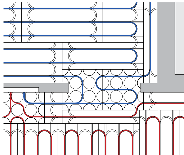
Výřez z instalačního schématu dveří
