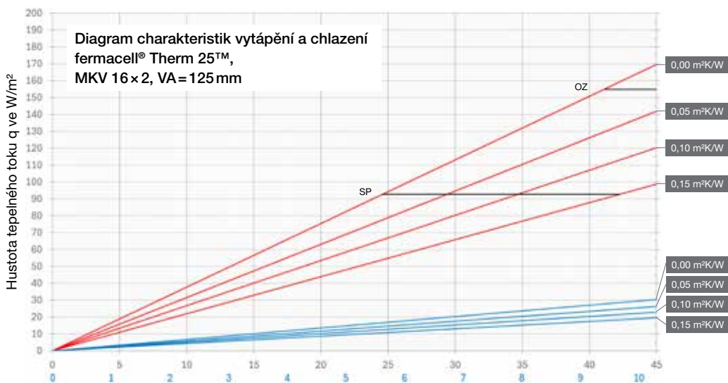
Lineární teplotní spád | Lineární teplotní spád (chlazení) v K SP: společné prostory | OZ: okrajová zóna
