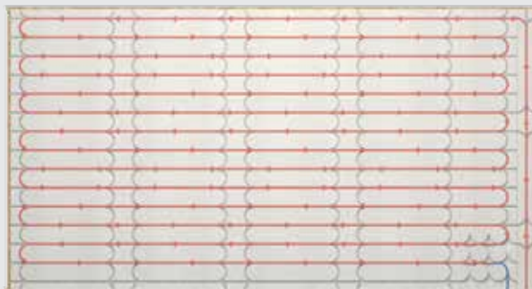
Pokládka topných trubek (16 mm)
